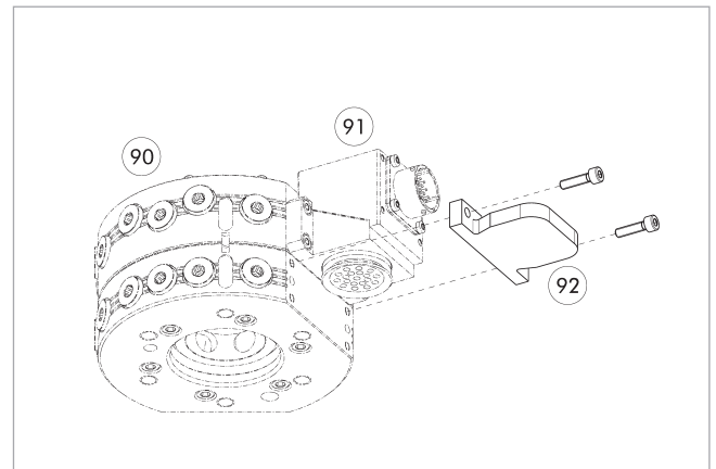
⑨④ 자동 톨 교환기 CPS
