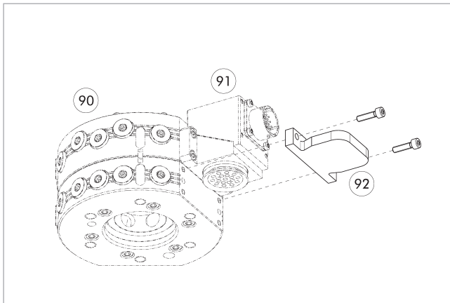
⑨④ 자동 툴 교환기 CPS
