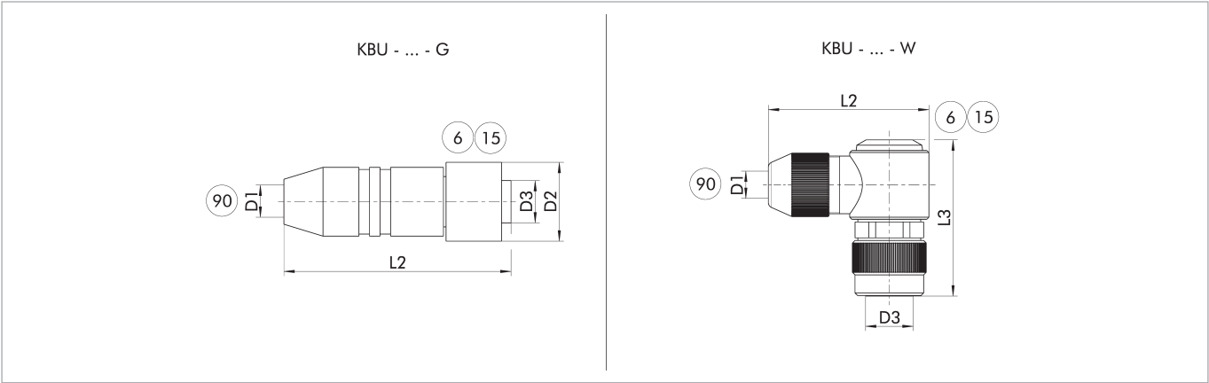
KBU - ... - G 직선형 출구가 있는 소켓 6 연결 모듈측 90 D1 - 최대 직경 연결 케이블 KBU - ... - W 각형 출구가 있는 소켓 15 소켓
