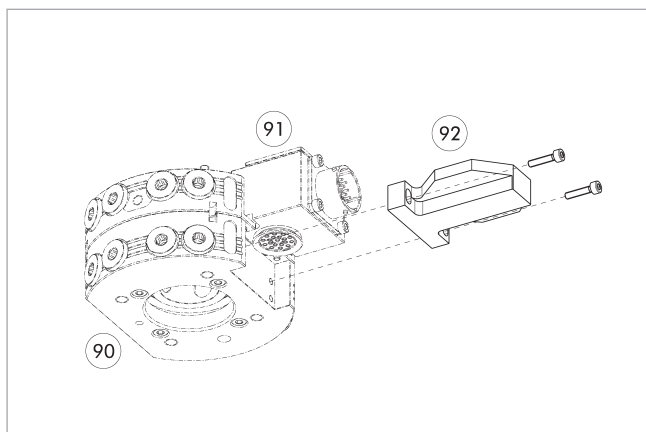
⑨⑩ 자동 툴 교환기 CPS
