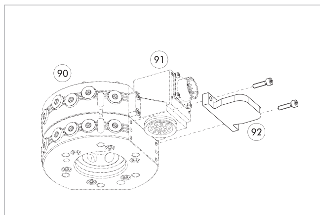
⑨0 자동 툴 교환기 CPS
